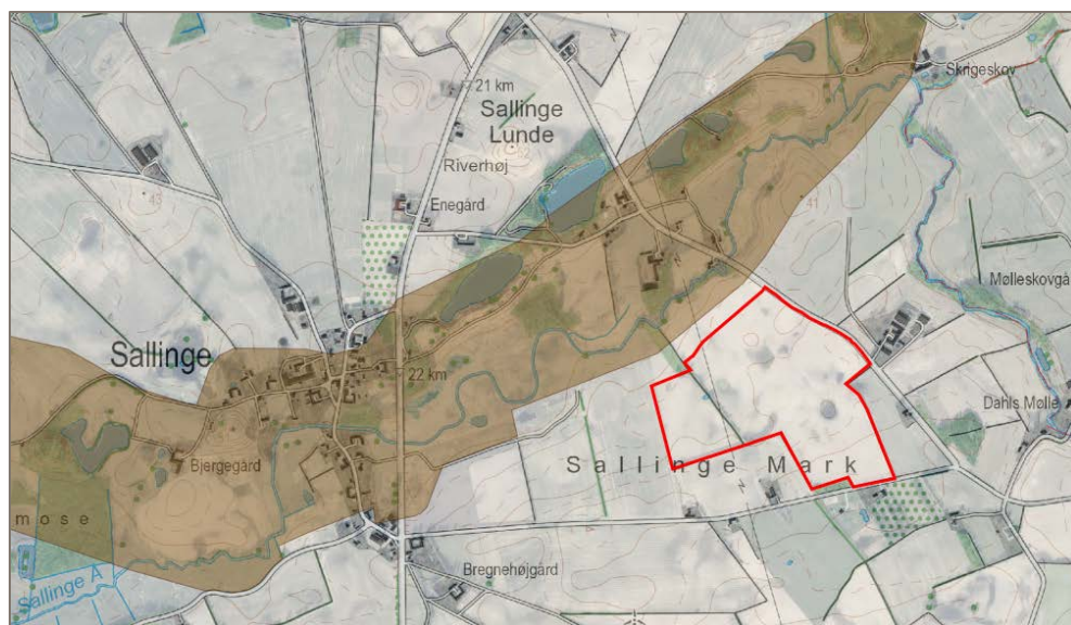
Figur 4-5 Planområdets beliggenhed i sammenhæng med område med geologiske bevaringsværdier (brun).
