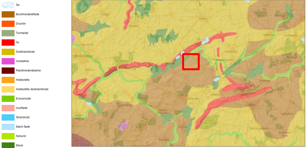
Figur 4-3 Geomorfologi. Planområdet (rød markering) ligger primært på moræneflade. Kilde: GEUS.
